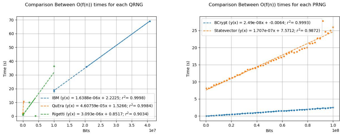
Figura 6: Ajuste lineal de las complejidades para cada RNG. Ibex no se pudo verificar por el coste de los shots, pero se espera también una complejidad lineal.
