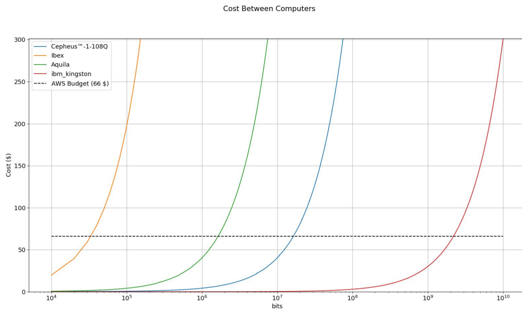
Figura 7: Comparación de las funciones costo. Eje x en escala logarítmica.
