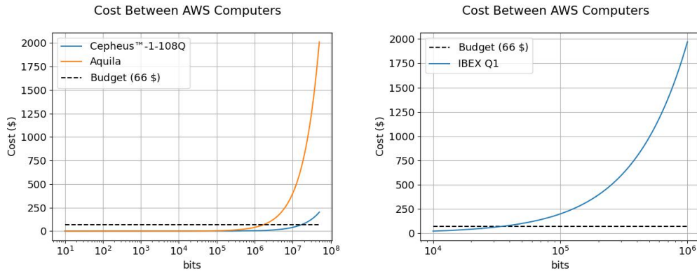
Figura 4: Comparación de las Funciones Costo de los computadores de AWS.
