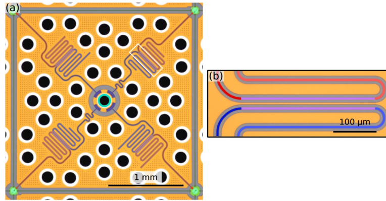
Figura 9: (a): Ejemplo del hardware para cuatro transmones (esquinas verdes). El dispositivo de medida es compartido y se encuentra en el centro de la placa[92].
