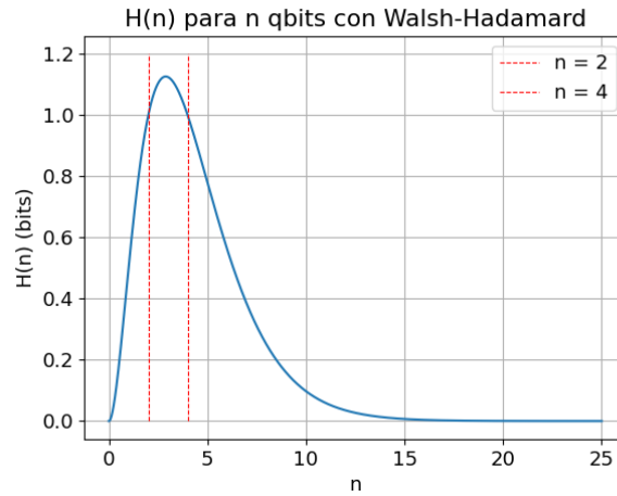
Figura 5: Entropía de Walsh-Hadamard para n qubits. Es de la forma:
